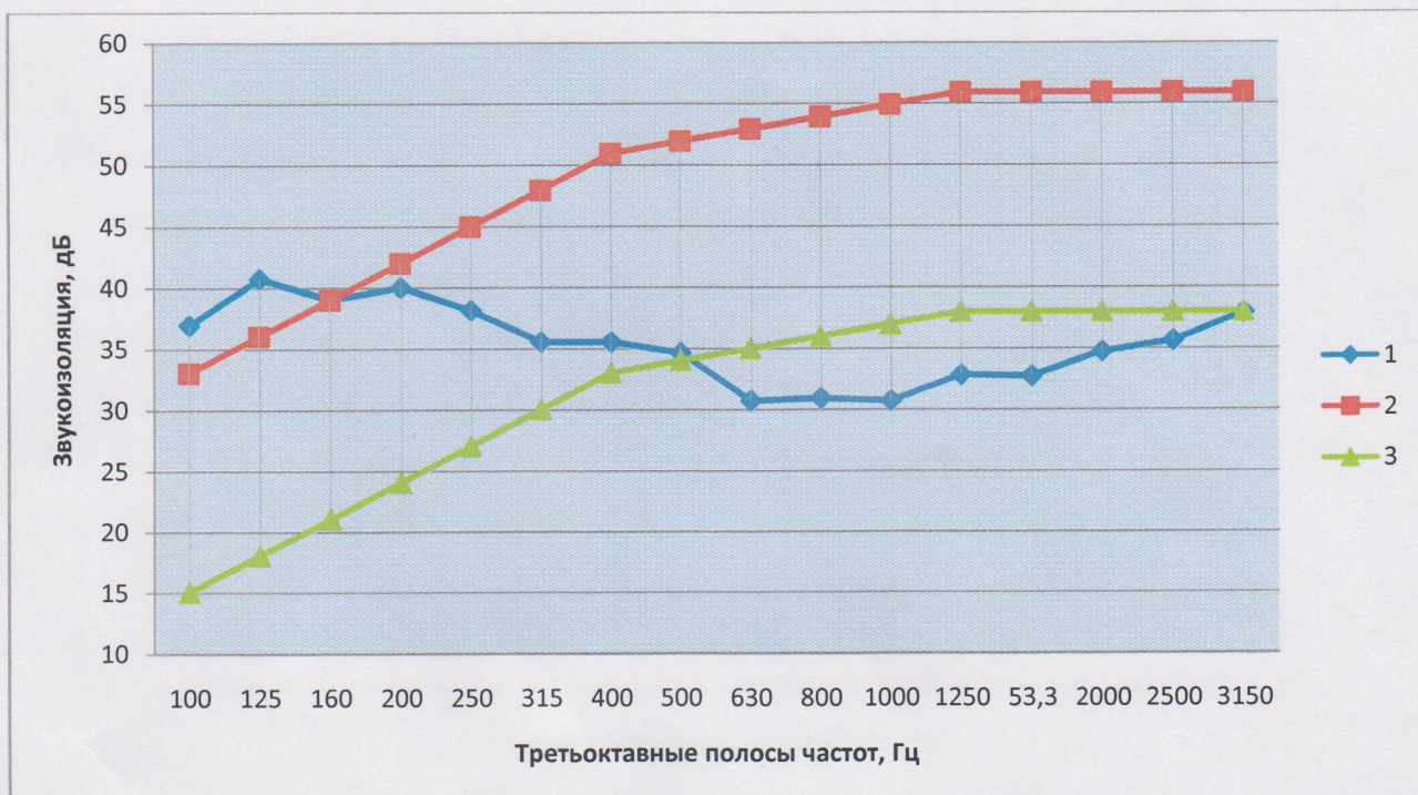
Рисунок 1. Частотная характеристика звукоизоляции
